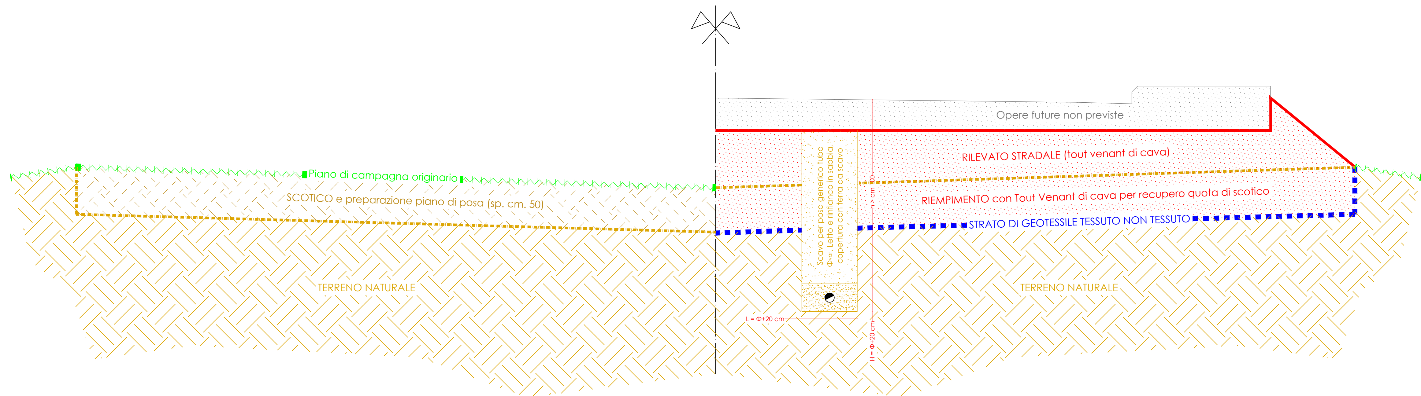
SEZIONE STRADALE TIPO IN STERRO - scala 1:20
